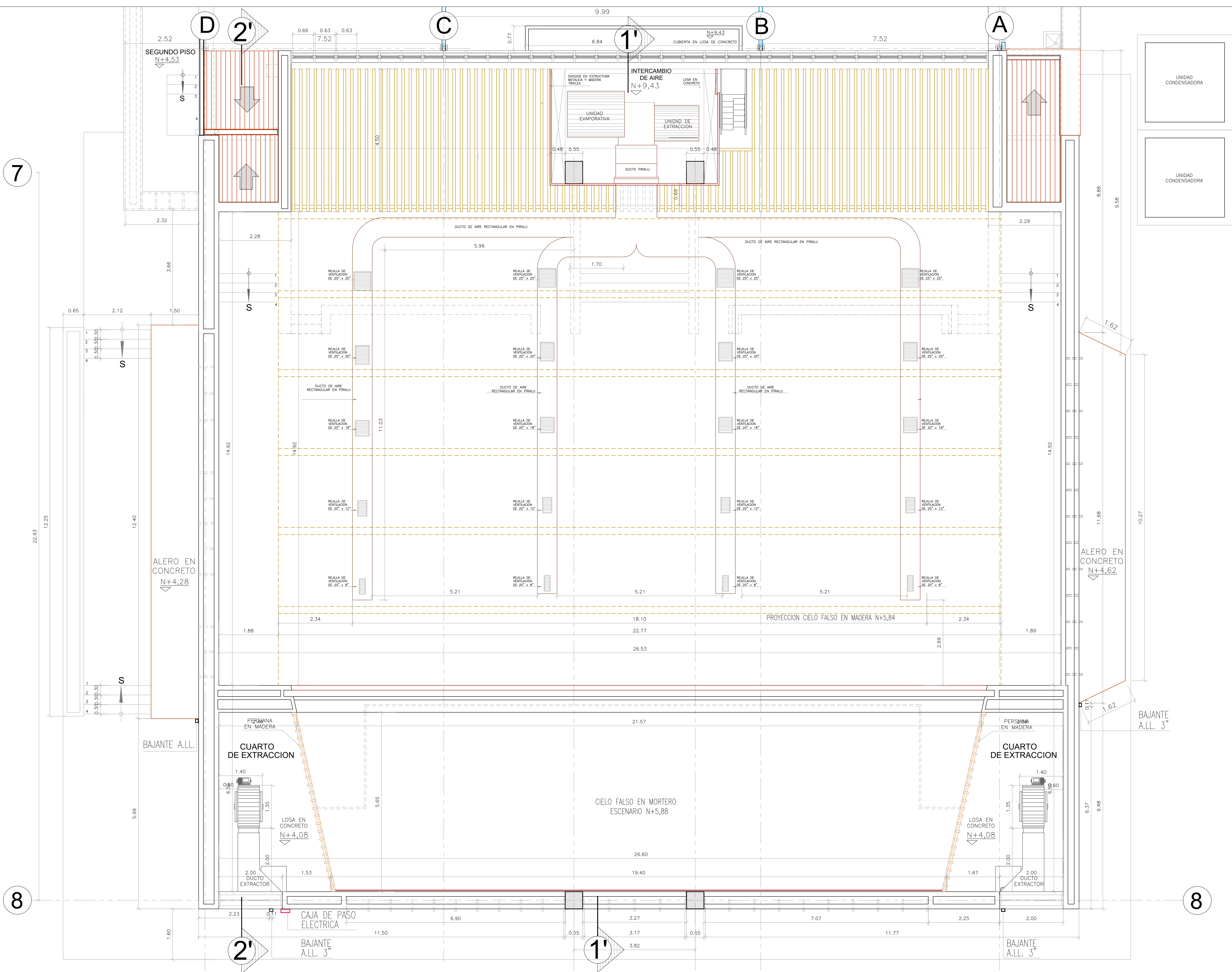
PLANTA DE LOCALIZACION DE LOS DUCTOS DE SUMINISTRO DE AIRE
